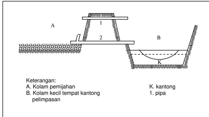
Gambar 4.20. Kolam pemijahan cara Kantong (Sumantadinata, 1983).
