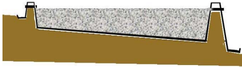
Gambar 2.18. Kemiringan dasar kolam
