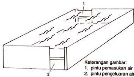
Gambar 2.21. Pintu pengeluaran dan pemasukan air berada disudut
