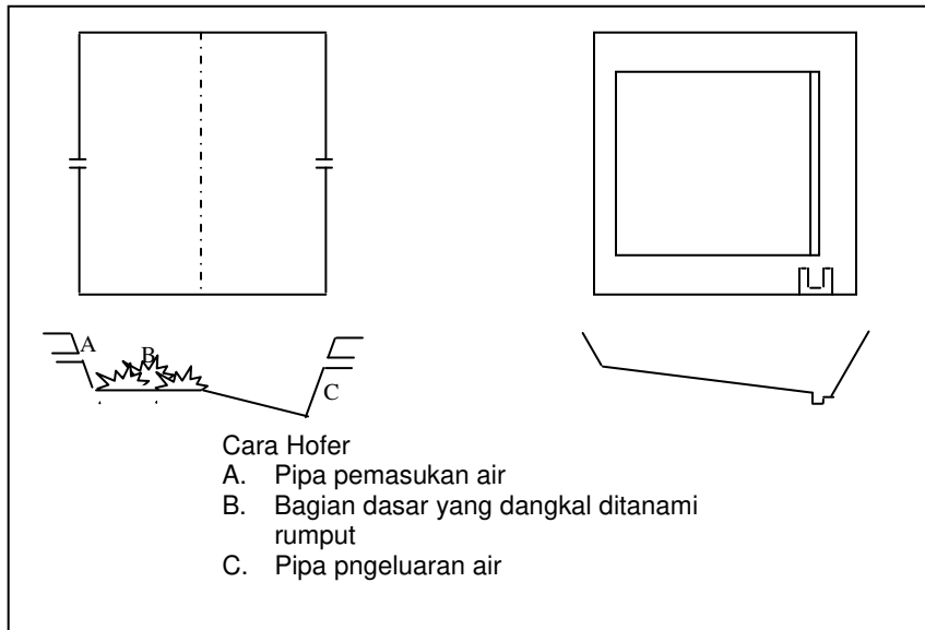
Gambar 4.22. Kolam pemijahan cara Hofer (Sumantadinata, 1983)
