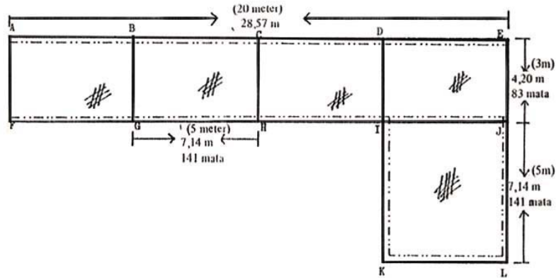
Gambar 2.35. Pola jaring
