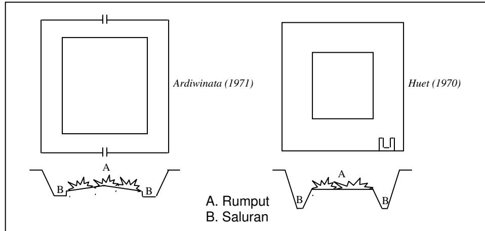
Gambar 4.21. Kolam pemijahan cara Dubisch (Sumantadinata, 1983)
