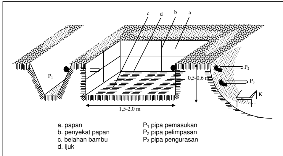
Gambar 4.19. Kolam pemijahan cara Magek (Sumantadinata, 1983).
